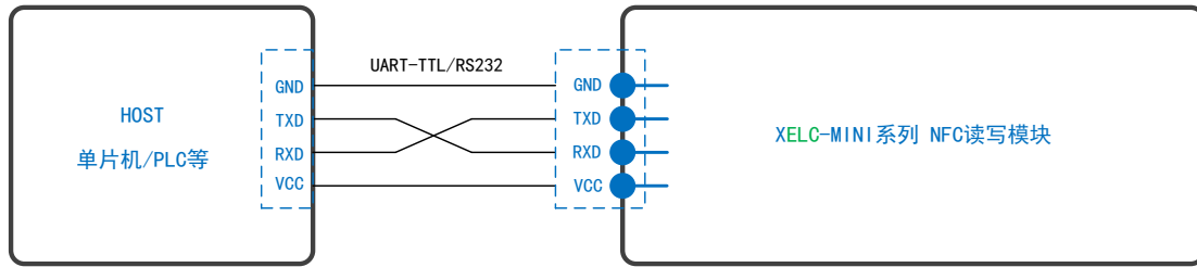
图 2.3 模块典型连接示意图
