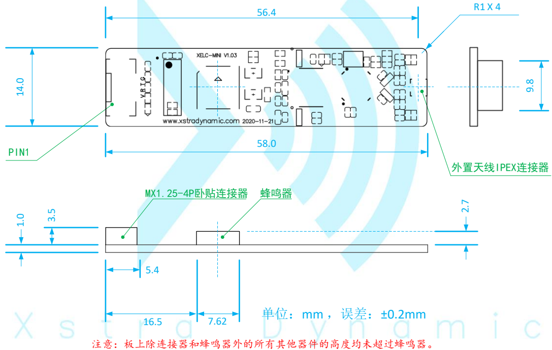
图 1.2 XELC-MINI 系列 NFC 读写模块机械尺寸
