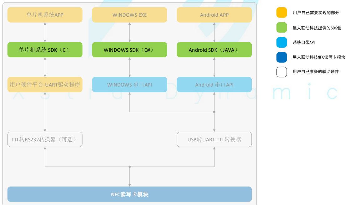
图 2.4 星人联动科技 NFC 读写卡模块 SDK 层次示意图
