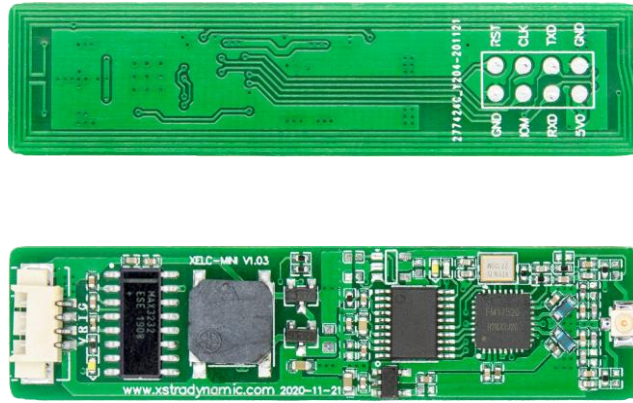
图 1.3 XELC-MINI 系列 NFC 读写模块 正（反）面图片
