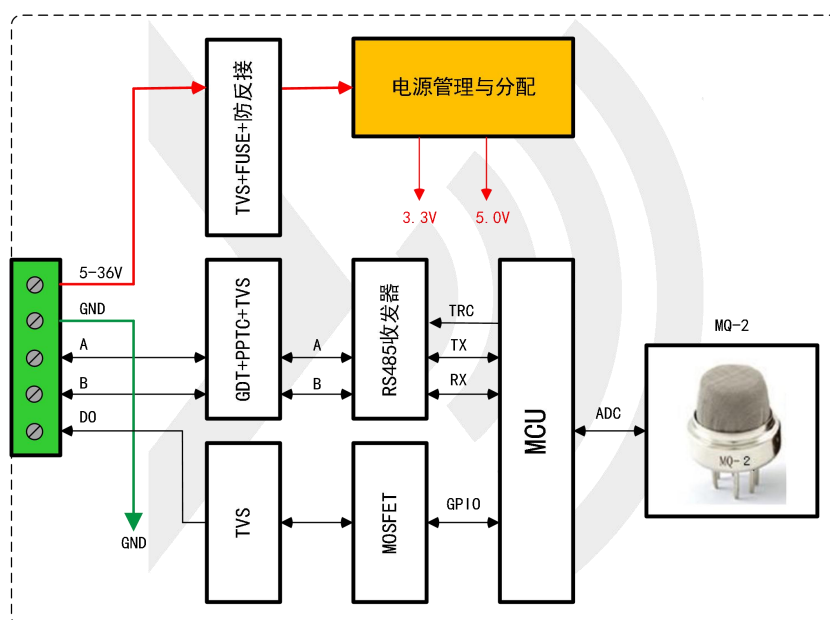
图 1.1 功能框图
