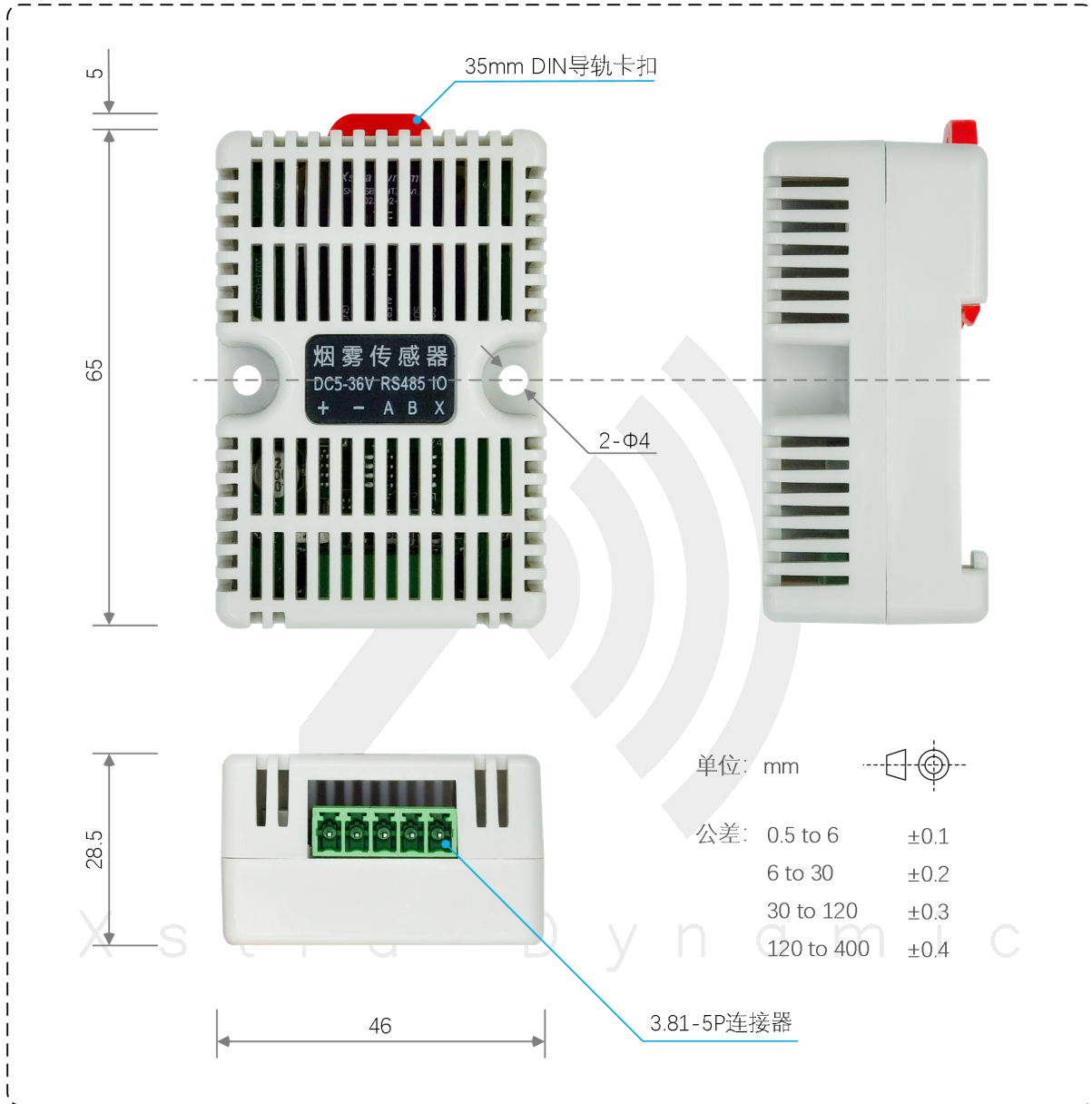
图 3.1 xSNS-MQ2 尺寸
